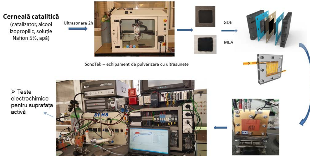
Linie de fabricare ansambluri MEA si testare PEMFC
